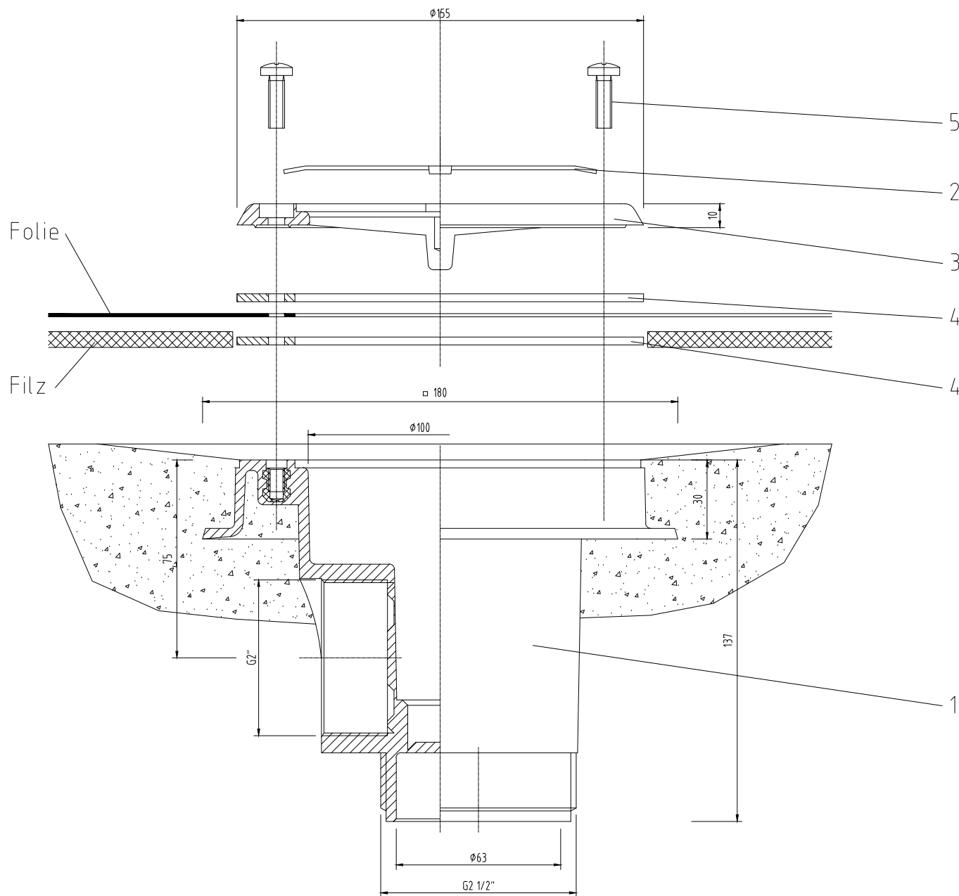
Bodenablauf ABS sw 2" mit Einlegerost Niro V4A 48140
