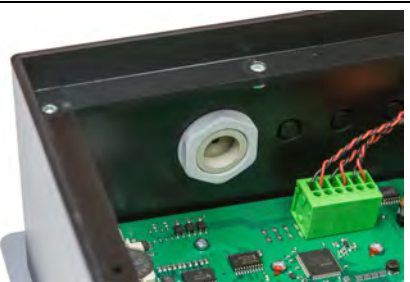
Befestigen Sie die Kabelverschraubung mit der zugehörigen Mutter ⑥
