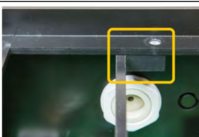
Drücken Sie die Montage-Schiene ② auf die Gewindeeinsätze im Pool Relax Gehäuse
